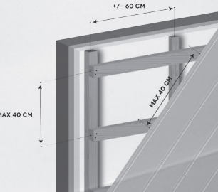
Schuine / diagonale plaatsing
